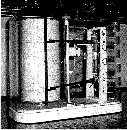
De thermohygrograaf; een apparaat dat de temperatuur en de luchtvochtigheid meet.
