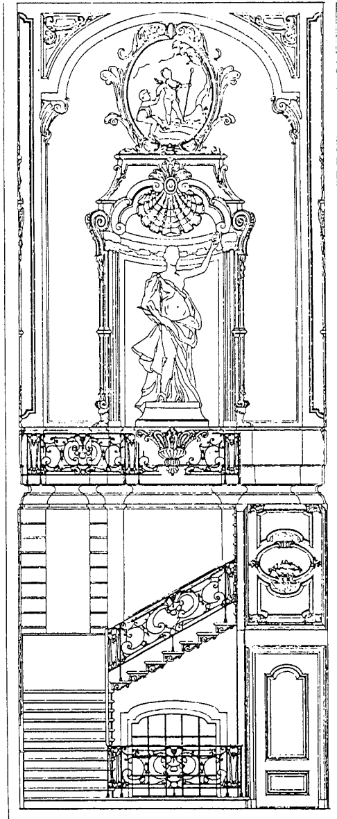
Trappenhuis van de Koninklijke Bibliotheek, in augustus 1940 opgemeten en getekend door R.D. Bleeker, in verband met dreiging van oorlogsschade.
