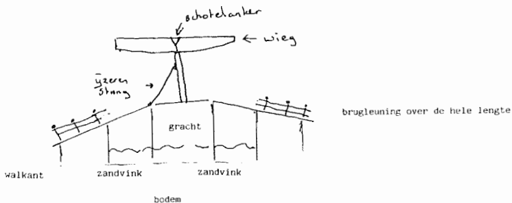
Een ruwe schets van de brug
